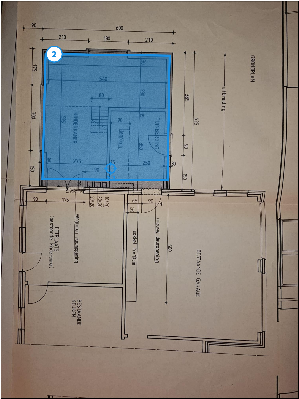
Legende van plan 1.7: Aanbouw - plafonds
