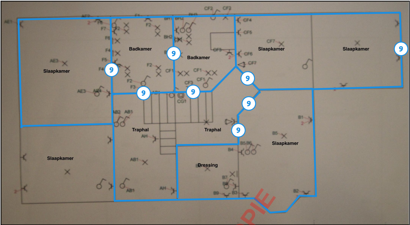
Legende van plan 1.12: 1ste verdiep
