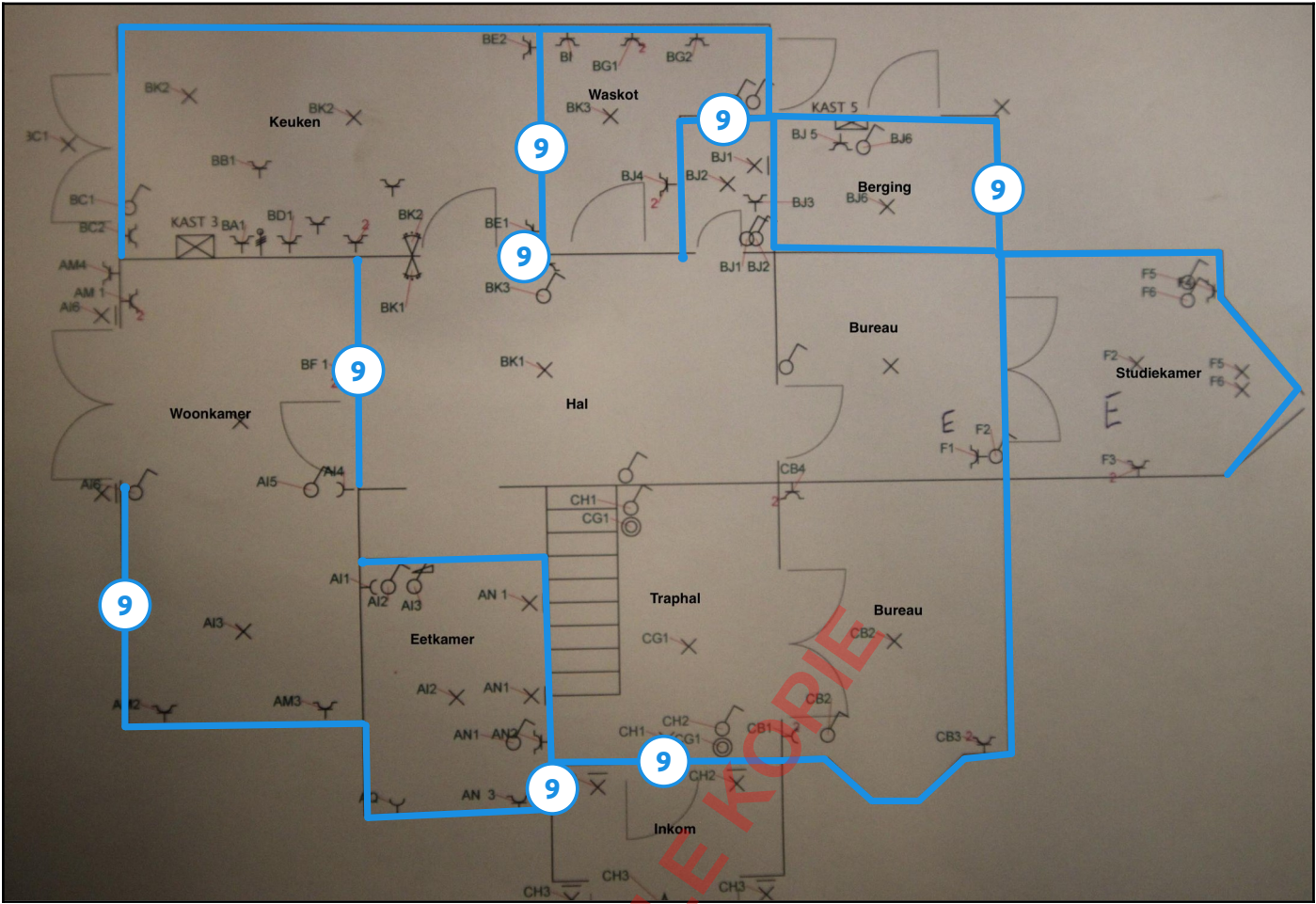
Legende van plan 1.11: Gelijkvloer
