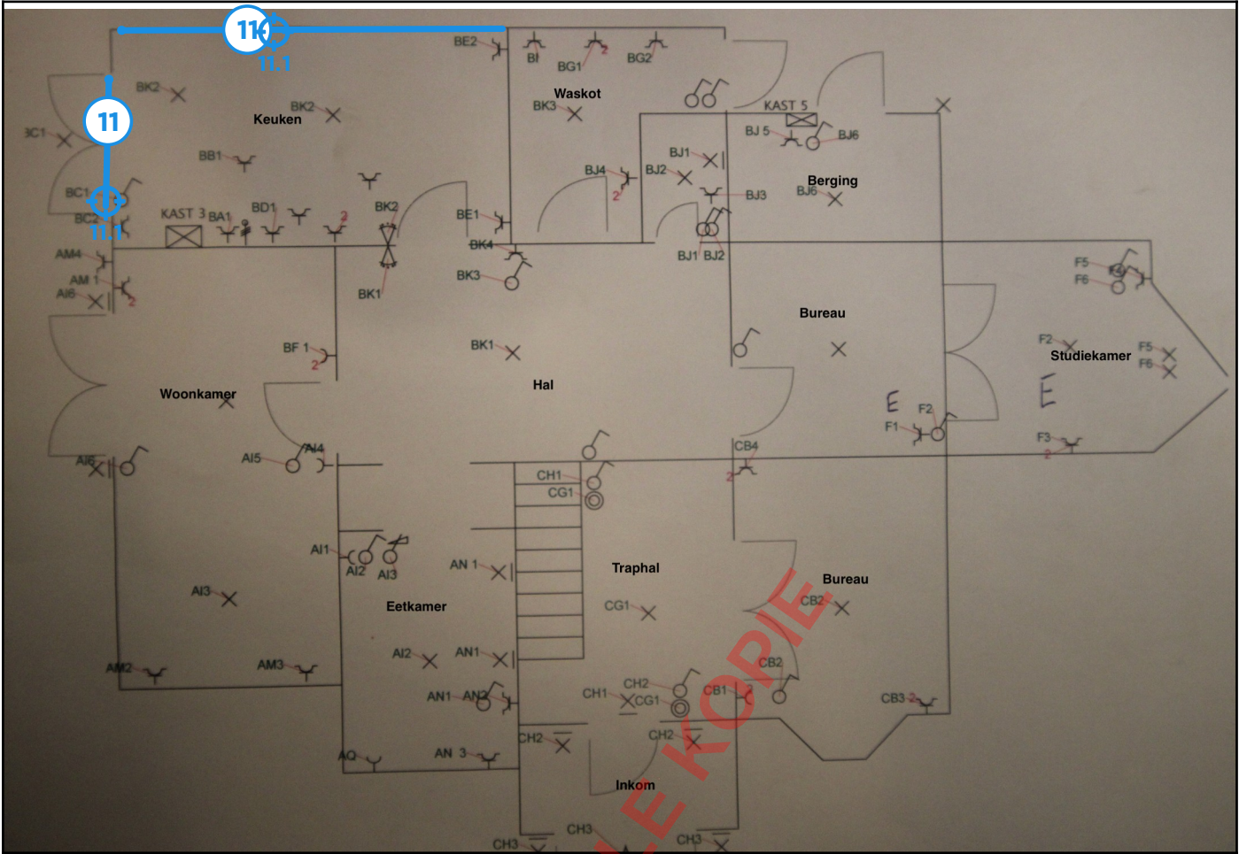
Legende van plan 1.7: Gelijkvloer
